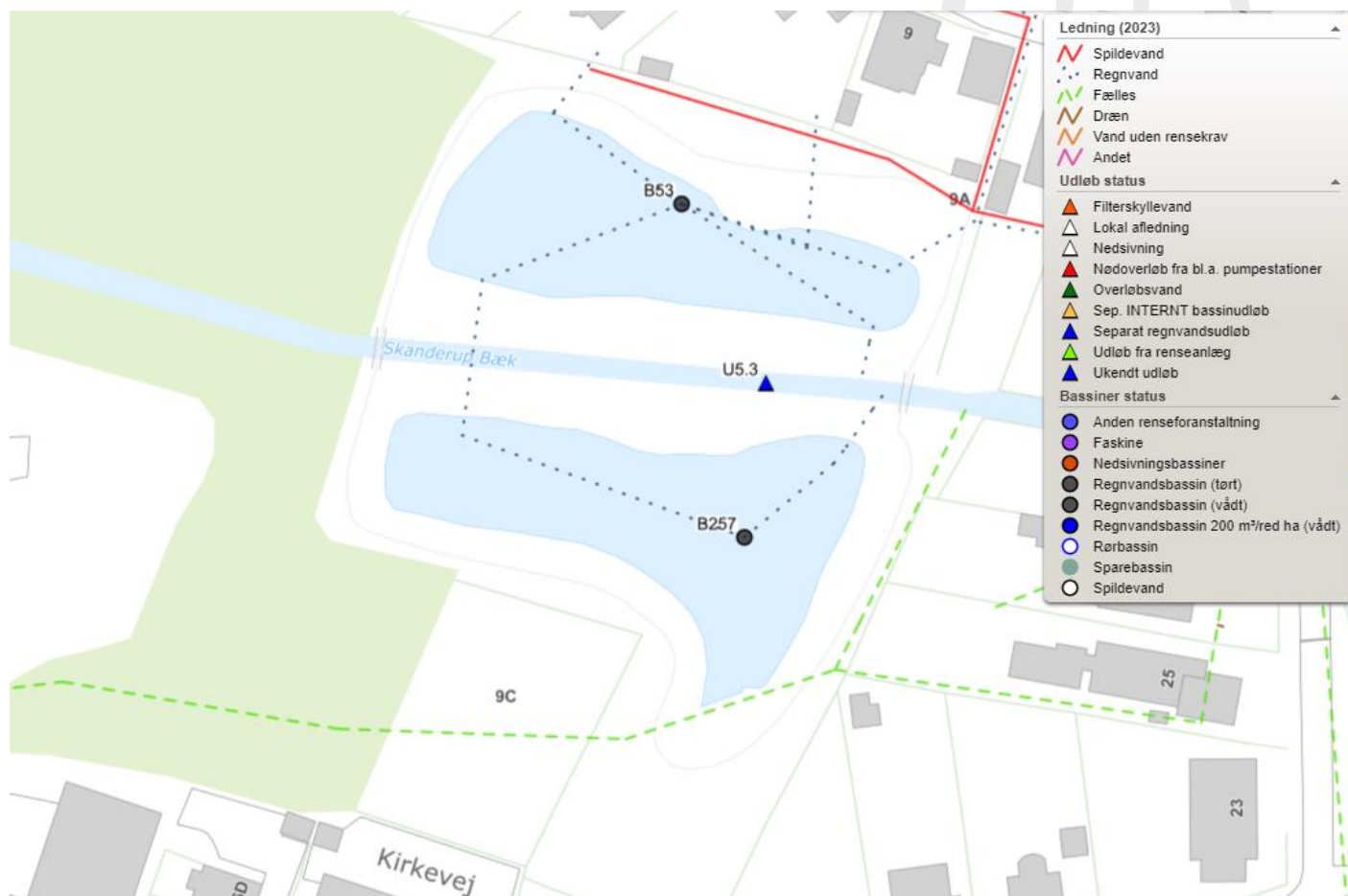
Figur 1. Nuværende placering af B53 samt udløbspunkt U5.3 til Skanderup Bæk. Nuværende placering af B257, som B53 fungerer som aflastningsbassin for, er også vist. Der indgår ligeledes en oversigt over diverse kloakledninger i og omkring bassinerne.
